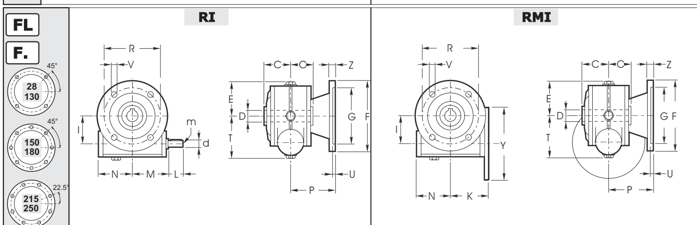
Dimensions générales / Dimensiones generales / Dimensões gerais
